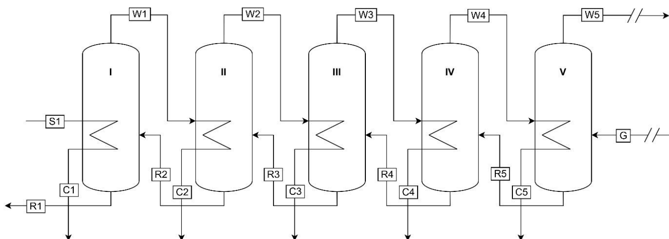
Obr. 2 Schéma päťstupňovej protiprúdnej odparky na čierny lúh.
